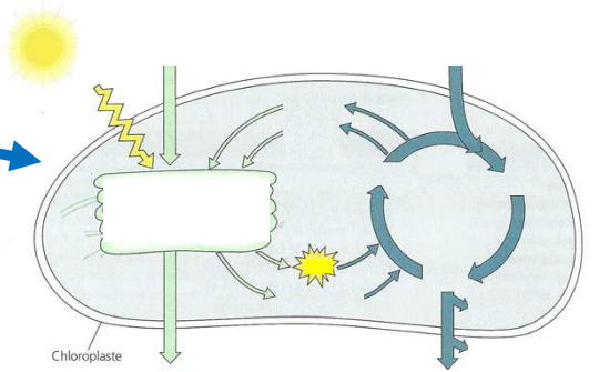
▲ Photosynthèse (dans les chloroplastes)
