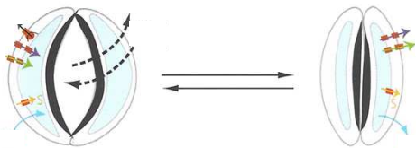
◀ Contrôle du flux hydrique par la plasmolyse/turgescence des cellules stomatiques : modèle simplifié
