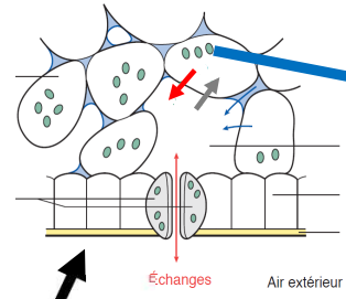
▲ Échanges entre la feuille et l'atmosphère (en journée)
