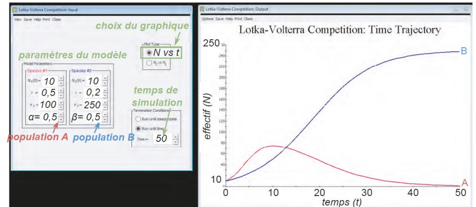
Figure TP12.3 Simulation d'une compétition interspécifique ( logiciel Populus ).
