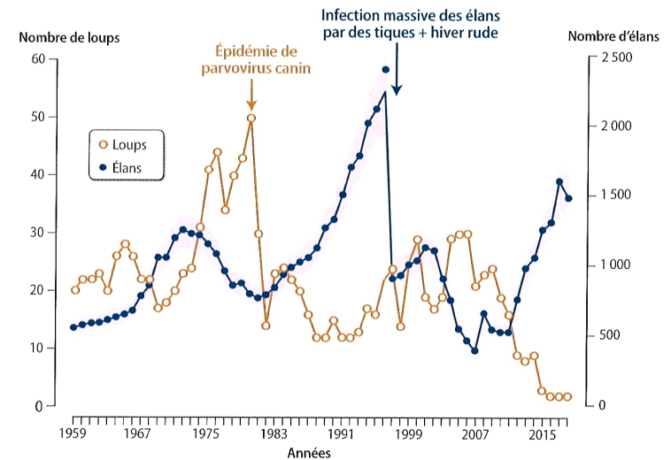
Figure A. Les fluctuations des effectifs d'élan et de loups dans le parc national de l'Isle Royale entre 1959 et 2018.
