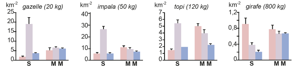
Figure 16.16 Densités (en nombre par km 2 ) des populations de 4 espèces d'herbivores.
