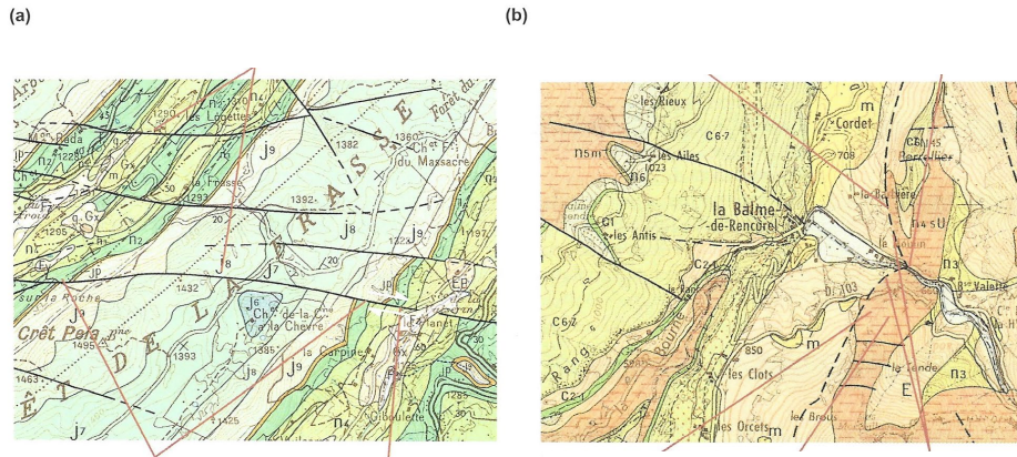
▲ FIGURE 17. Typologie des failles : une vision plus complète. D'après PEYCRU et al. (2015)
