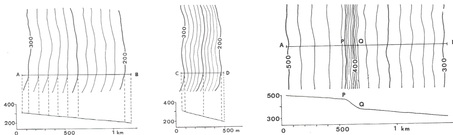
FIGURE b. Pentés régulières. D'après FOUCAULT & RAOULT (1975)
