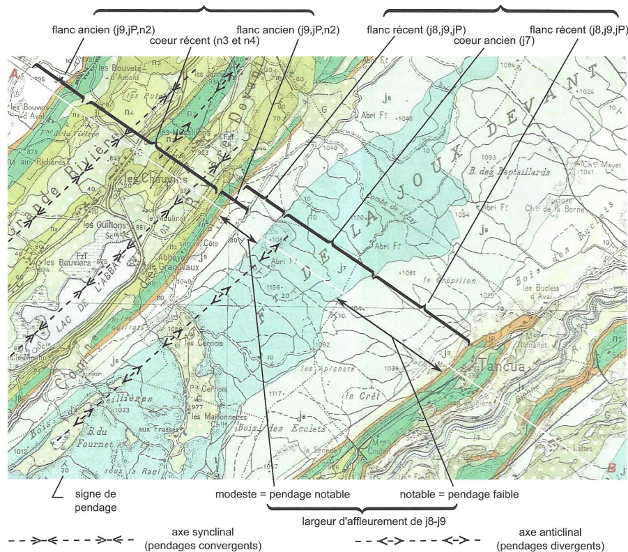
▲ FIGURE 20. Anticlinal et synclinal . D'après EMMANUEL et al. (2007)
