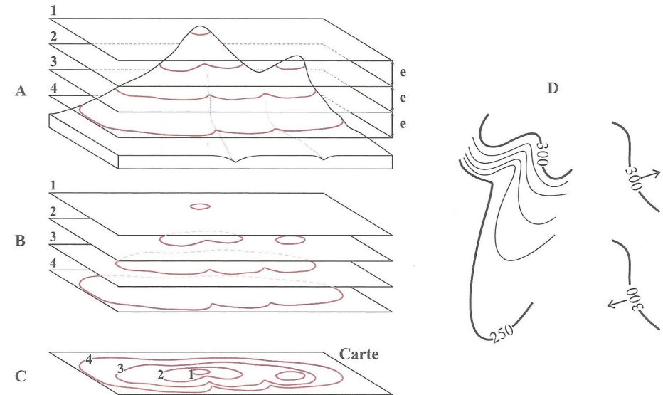
Les courbes de niveau.
