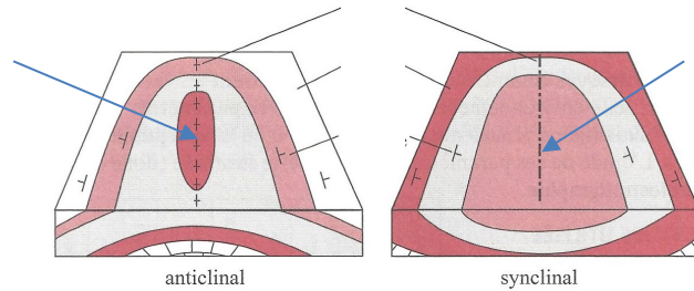
▲ FIGURE 20. Anticlinal et synclinal . D'après EMMANUEL et al. (2007)
