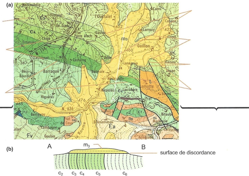
Une discordance en carte.
