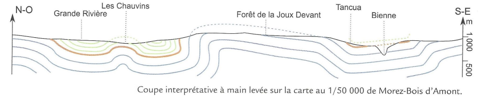
▲ FIGURE 22. Plis en coupe (profil AB de la figure 21) . D'après PEYCRU et al. (2015)
