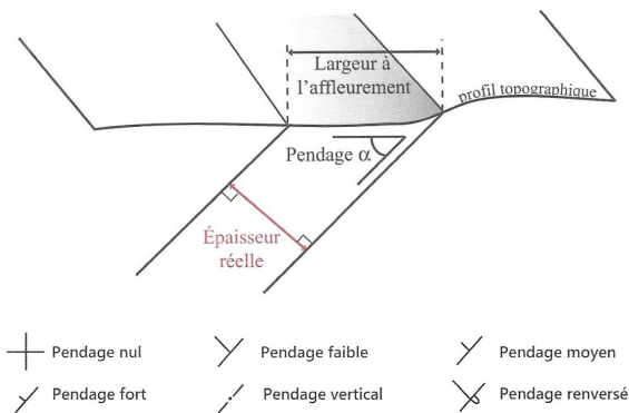
▲ FIGURE 6. Pendage et épaisseur d'une couche géologique. D'après EMMANUEL et al. (2007) et BORDI et al. (2018)
